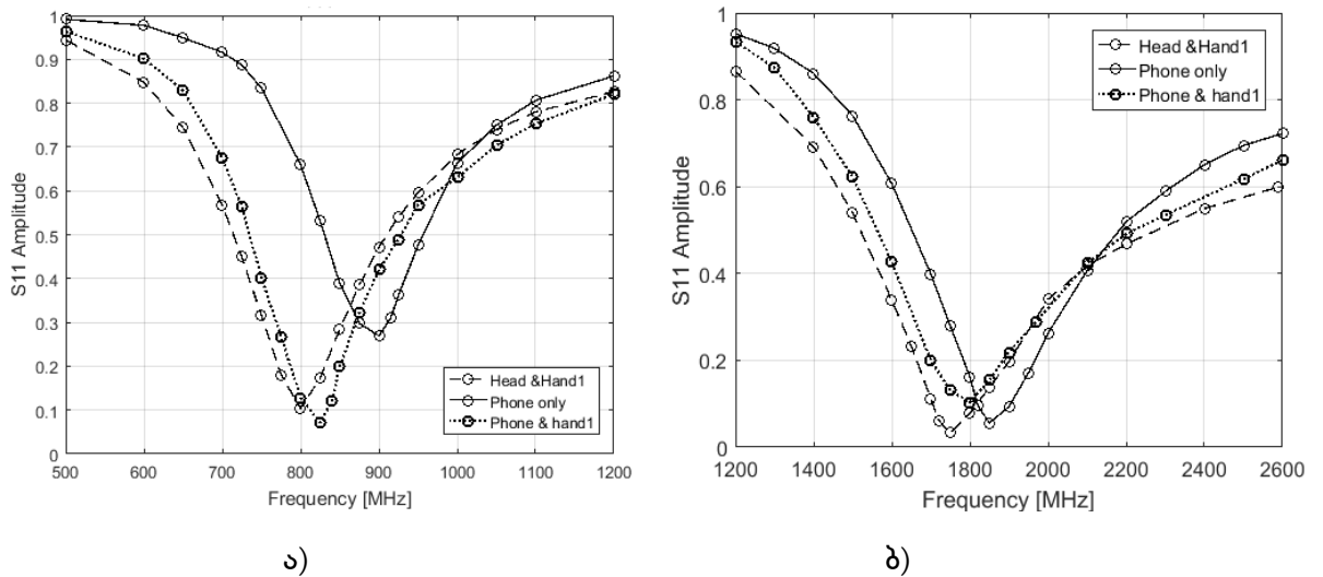
სურ 2.3. 2. დიპოლური ანტენის სიხშირული მახასიათებელი ა) 900 მჰც და ბ) 1900 მჰც სიხშირეებისათვის.
